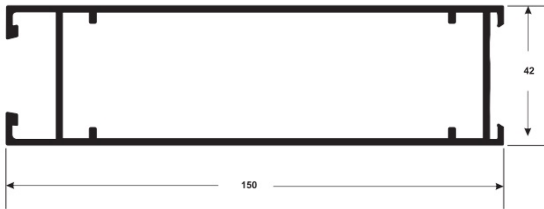
P-194 0,799 Kg/m
