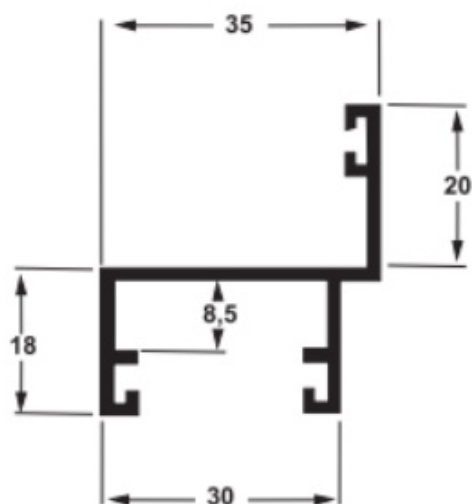
Y-140 0,406 Kg/m
