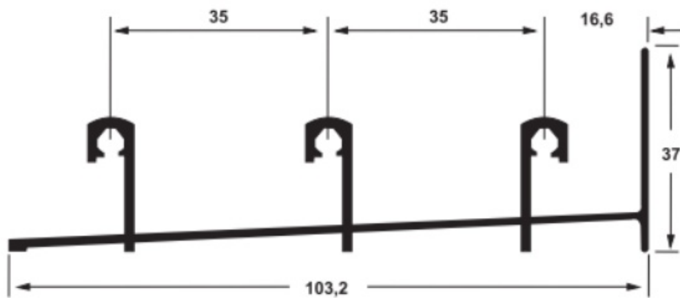
SU-230 0,954 Kg/m
