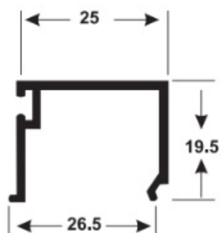
U-611 0,192 Kg/m
