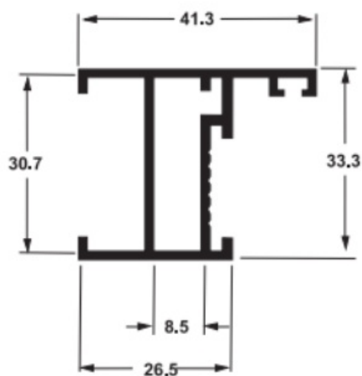
SU-279 0,565 Kg/m
