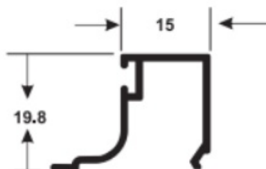
U-552 0,186 Kg/m
