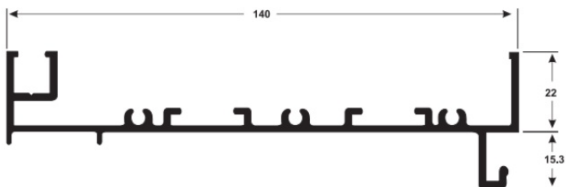
MN-001 1,377 Kg/m
