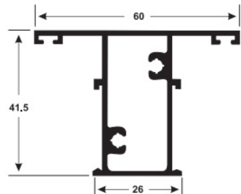
P-280 0,855 Kg/m
