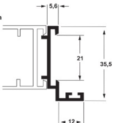
L-519 0,300 Kg/m
