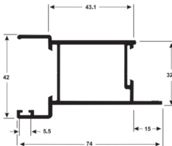
LG-059 0.169 Kg/m
