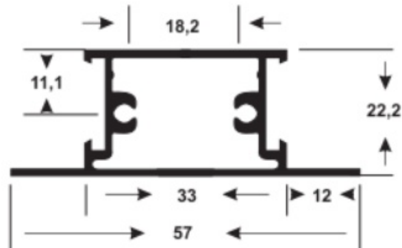
SU-227 0,550 Kg/m
