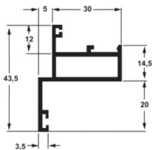
P-120 0,535 Kg/m
