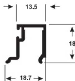
LG-026 0.158 Kg/m
