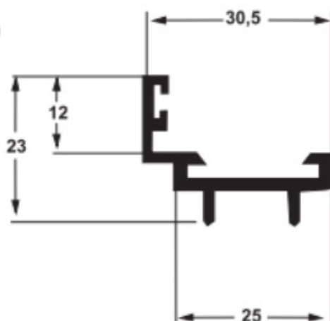
L-715 0,298 Kg/m
