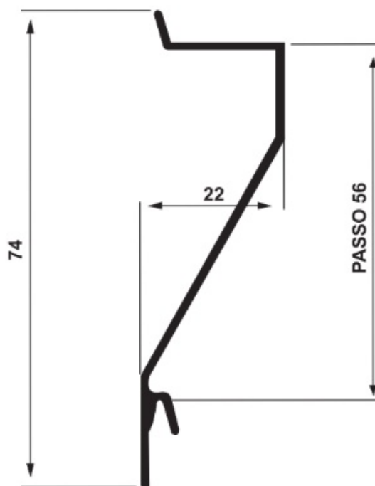
Z - 203 0,301 Kg/m
