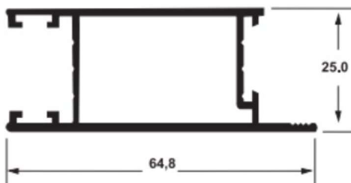
SU-245 0,634 Kg/m
