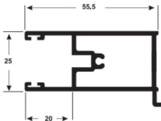
MN-007 0,710 Kg/m
