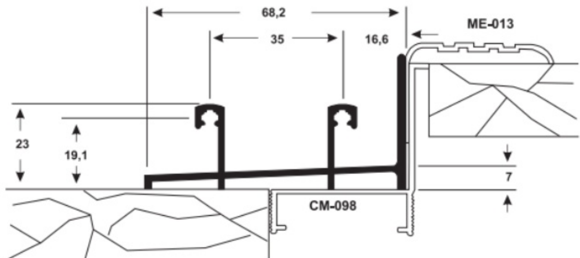
SU-230 0,954 Kg/m
