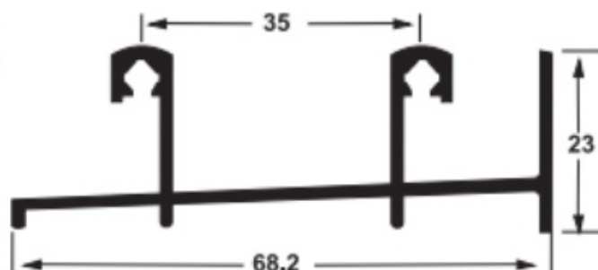
SU-260 0,631 Kg/m
