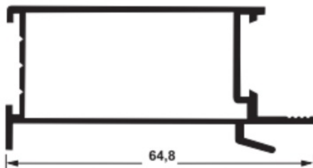
SU-243 0,620 Kg/m
