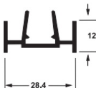
SU-291 0,263 Kg/m
