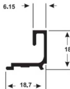
LG-027 0.149 Kg/m
