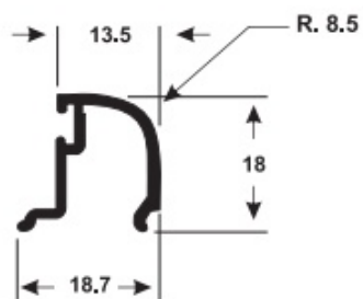
LG-026 0.158 Kg/m
