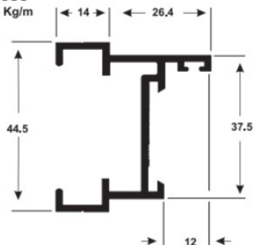
LG-056
