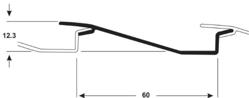
VZ - 051 0,268 Kg/m
