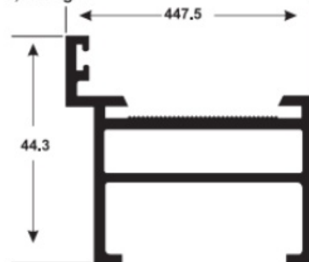
P-280 0,855 Kg/m
